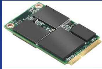
SSD 熱固膠 (SSD underfill)
